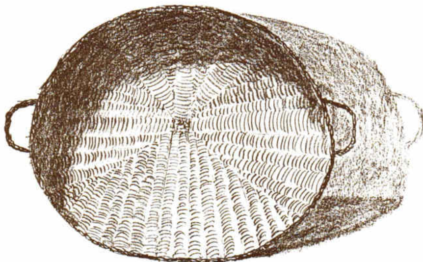
'n Wanne
