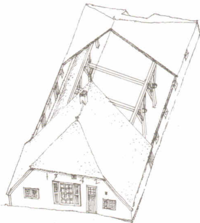
Afb. 2 Bouwtekening Erve Zeysveld (2).
