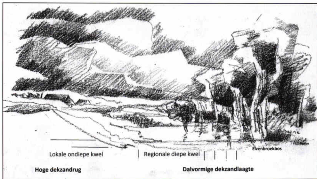
Afb. 4: Het ontstaan van kwel in een dekzandlaagte.
