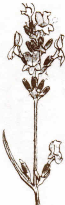
Lavendel ( lavandula officinalis )
